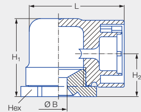
Type 302.6xx.51.KB
